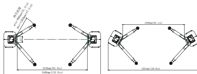
对称安装
